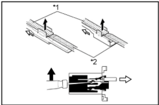
⇨ 拉起 ➡ 拉出 *1 锁止卡子 *2 专用工具
