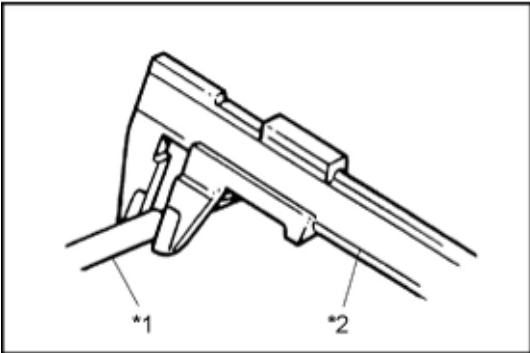
线束外径
