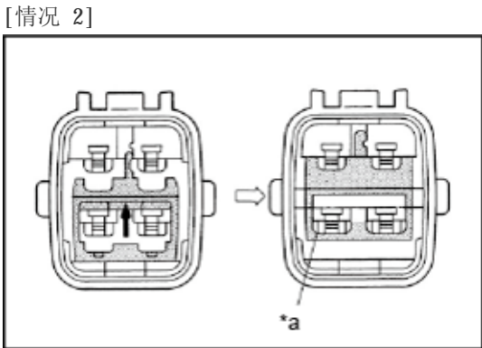
*a 完全锁止位置
