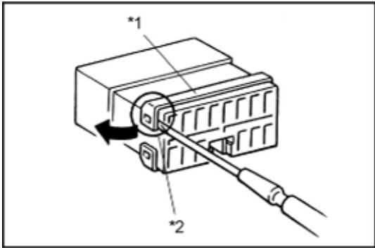
*1 固定架 *2 侧锁
