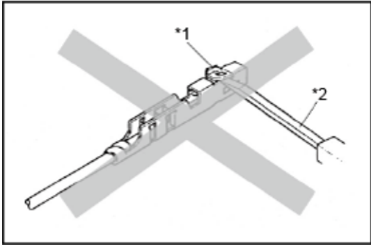
绝缘置换型连接器
