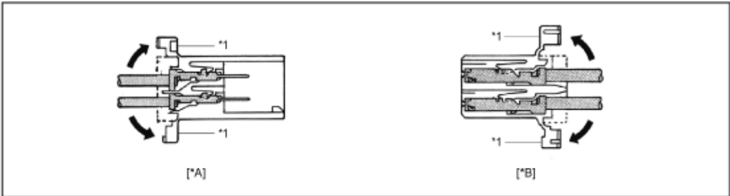
*1 凸耳
