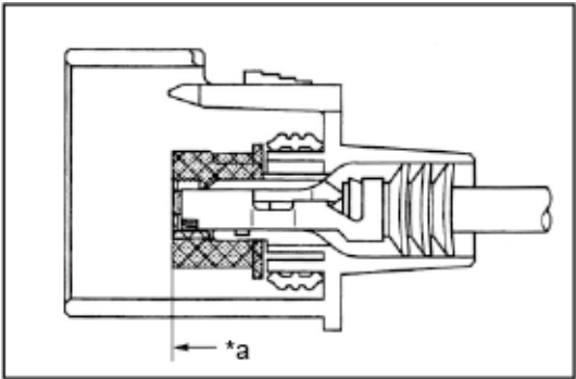
[情况 1]
