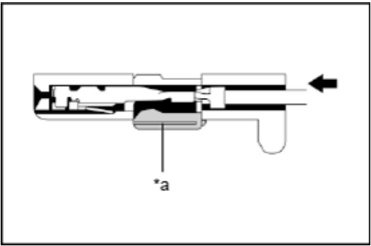
*a 临时锁止位置
