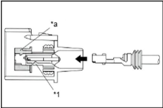
*1 端子锁止卡子 *a 端子固定架在临时锁止位置
