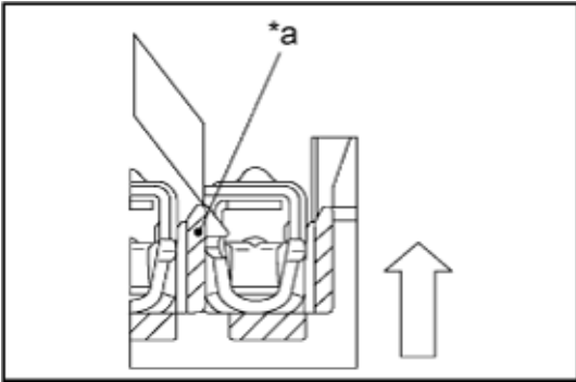
*a 推动时拉出端子
