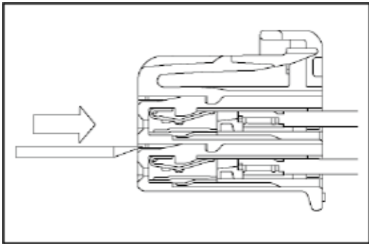
*1 夹具插入孔
