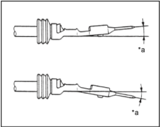
端子垂直方向弯曲
