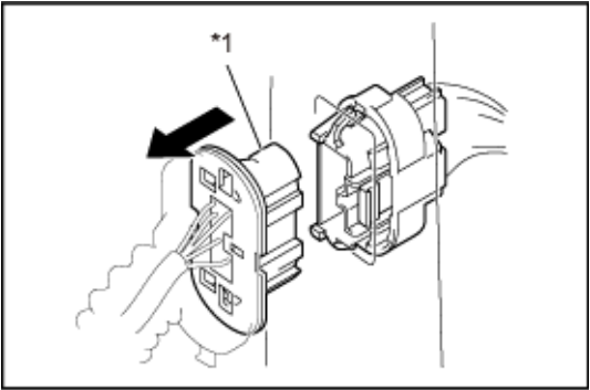
*1 插座式连接器
