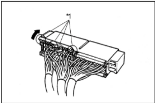
*1 凸耳
