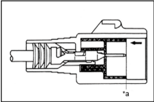
*a 完全锁止位置
