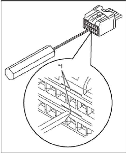
*1 夹具插入孔
