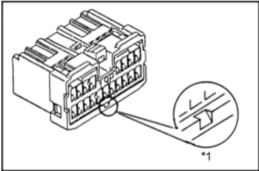
*1 检修孔
