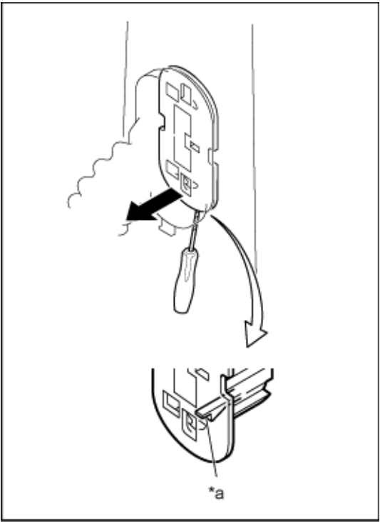
*a 工具插入点
