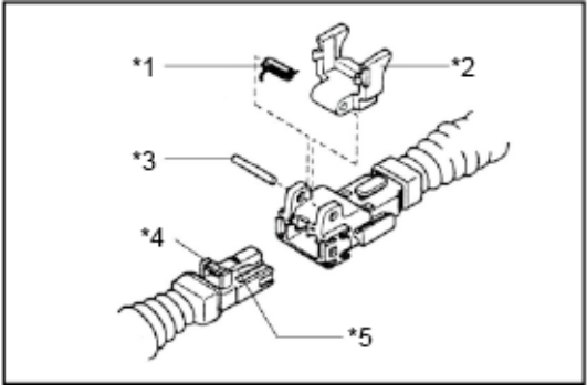
*1 螺旋弹簧 *2 双重锁止装置销 *3 销 *4 凸面部分 *5 主锁止装置
