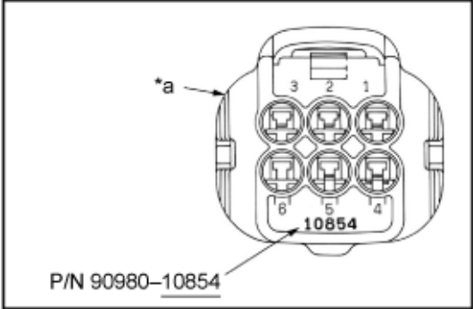
*a 连接器主体背面
